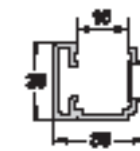
Οδηγός Ραμποτέ / Rabeté rail Κωδ. / Code F50-310 Βάρος / Weight 427 gr/m
