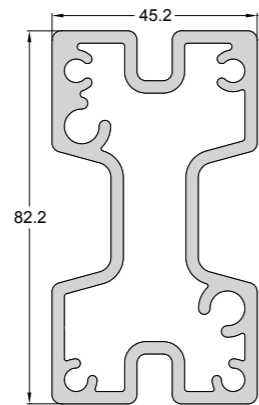
Σύνδεσμος κολώνας 2200-102 Connector for column 2200-102 Κωδ. / Code 2200-903 Βάρος / Weight 2758 gr/m
