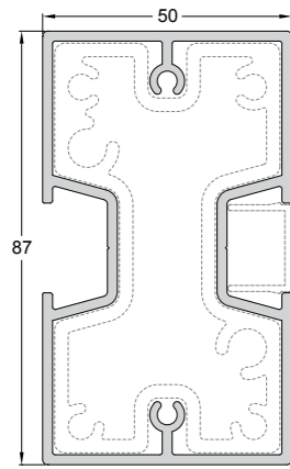
Κολώνα-Χώρισμα Column - Transom Κωδ. / Code 2200-102 Βάρος / Weight 1885 gr/m
